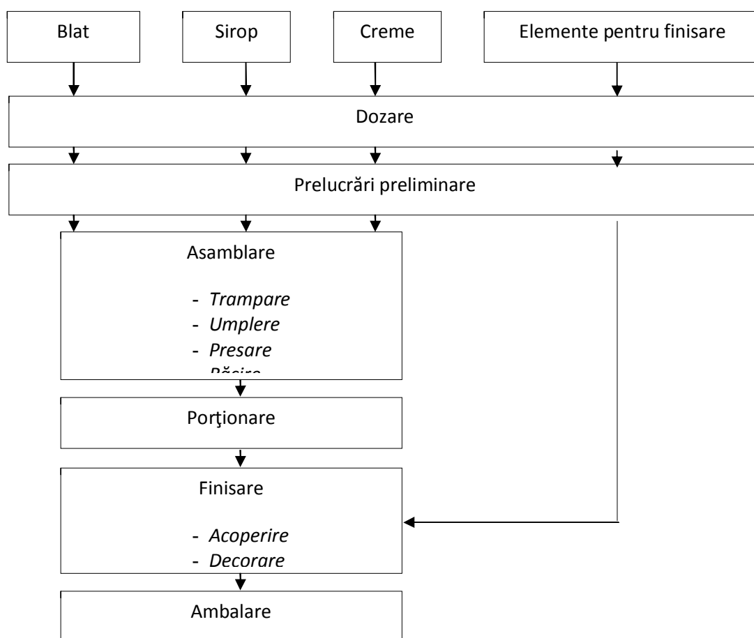
Schema nr. 5.1.3. Procesul tehnologic de obținere a prăjiturilor cu blat
