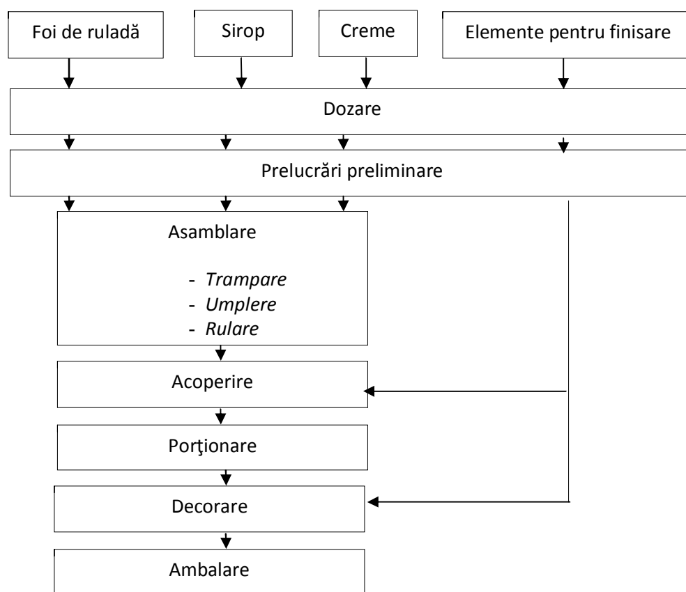
Schema nr. 5.1.4. Procesul tehnologic de obținere a prăjiturilor cu foi de ruladă
