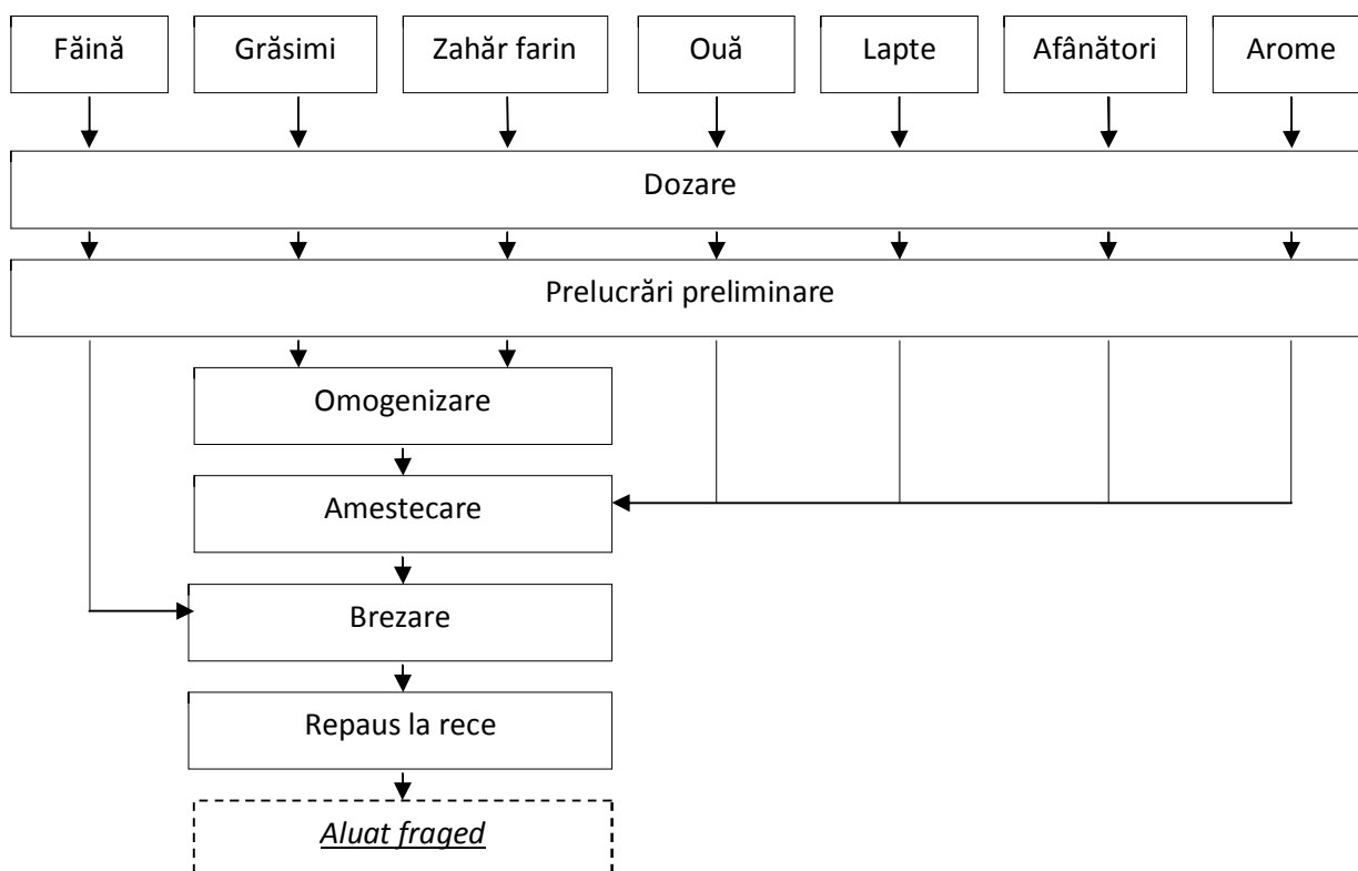
Fig. 3.4.3 Schema tehnologică de obținere a aluatului fraged frământat
