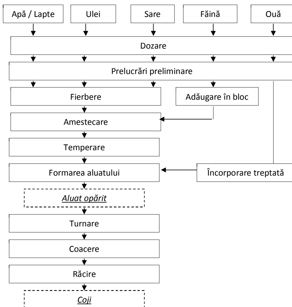
Fig. 3.3.3 Schema tehnologică de obținere a aluatului opărit
