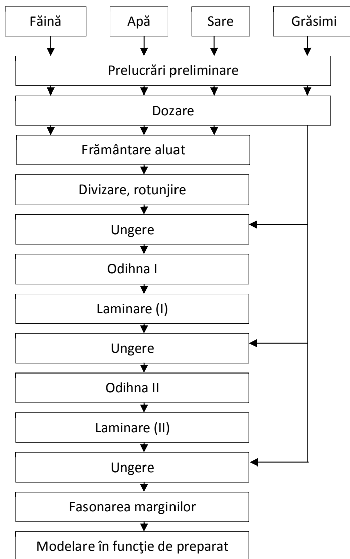
Fig.3.2.3. Schema tehnologică de obținere a foii de plăcintă românească
