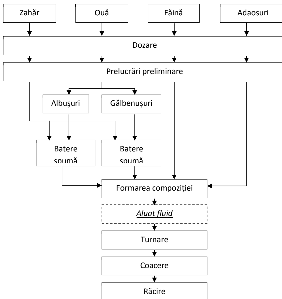
Fig. 3.5.3 Schema tehnologică de obținere a aluatului fluid
