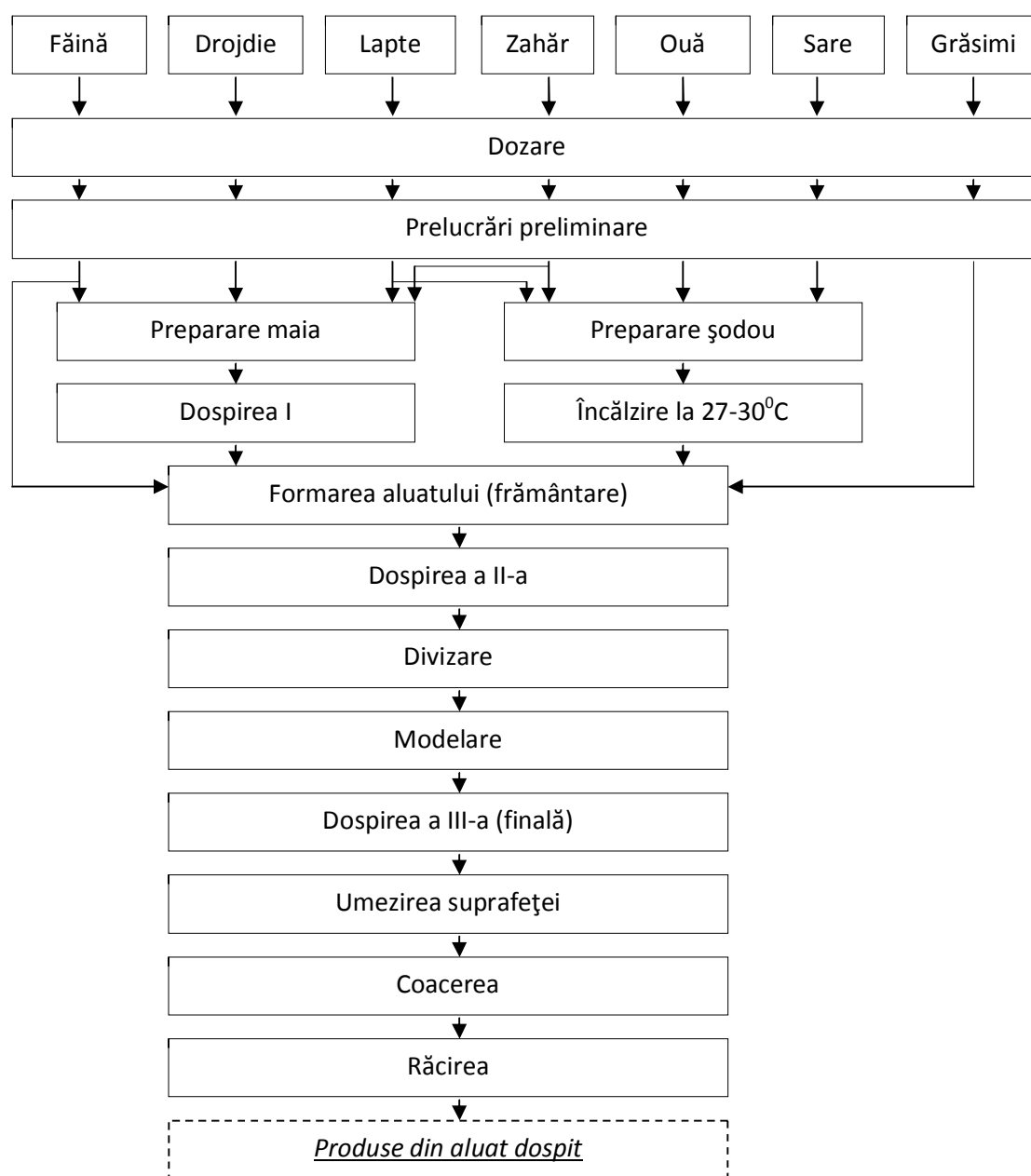
Fig.3.6.3. Schema tehnologică de obținere a preparatelor din aluat dospit (cu adaosuri)
