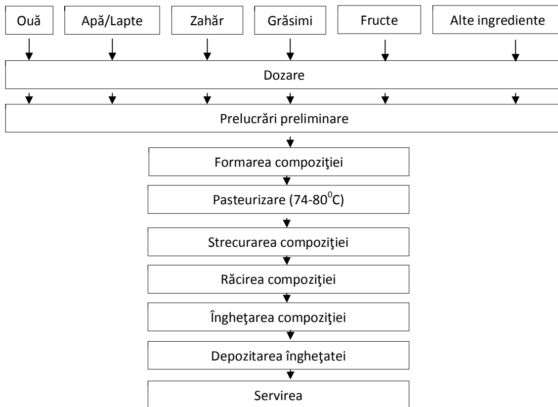
Fig. 6.3.3. Schema tehnologică generală de preparare a înghețatelor
